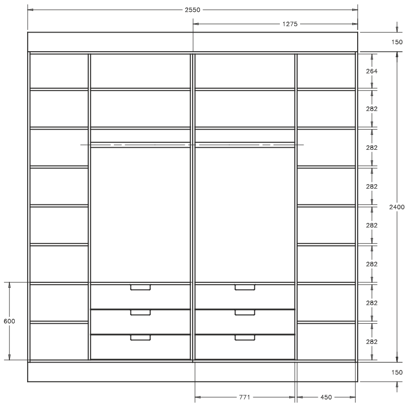
SKRIN ZOBRAZENA BEZ POSUVNYCH DVERI
