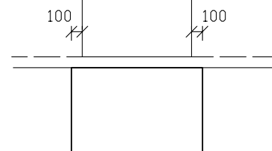
ZÁKLAD POD DVEŘNÍM OTVOREM - POHLED FUNDAMENT UNTER TÜRÖFFNUNG - ANSICHT
