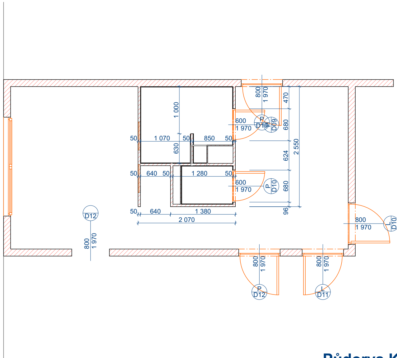
Půdorys Koupelny Stávající stav
