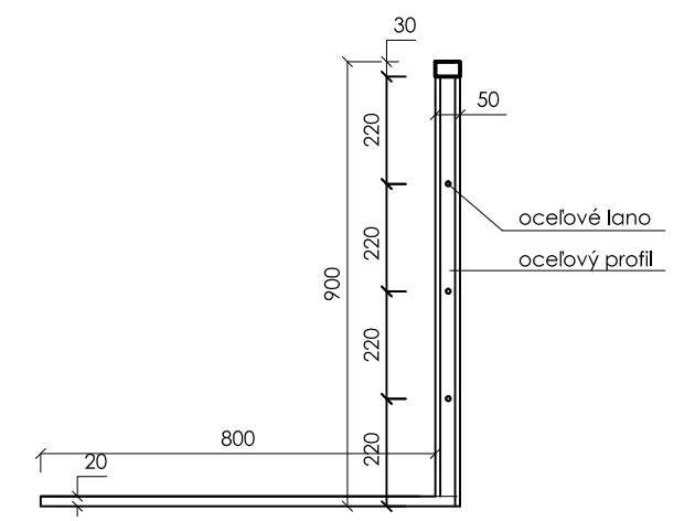
rez 1 - 1'
