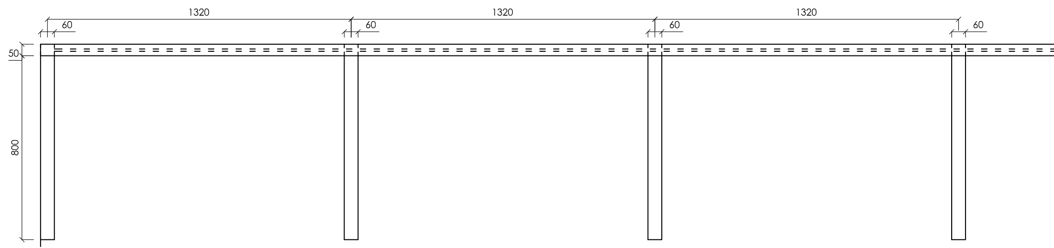
pôdorys zábradlia
