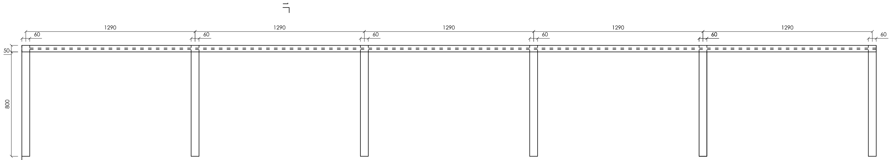
pôdorys zábradlia
