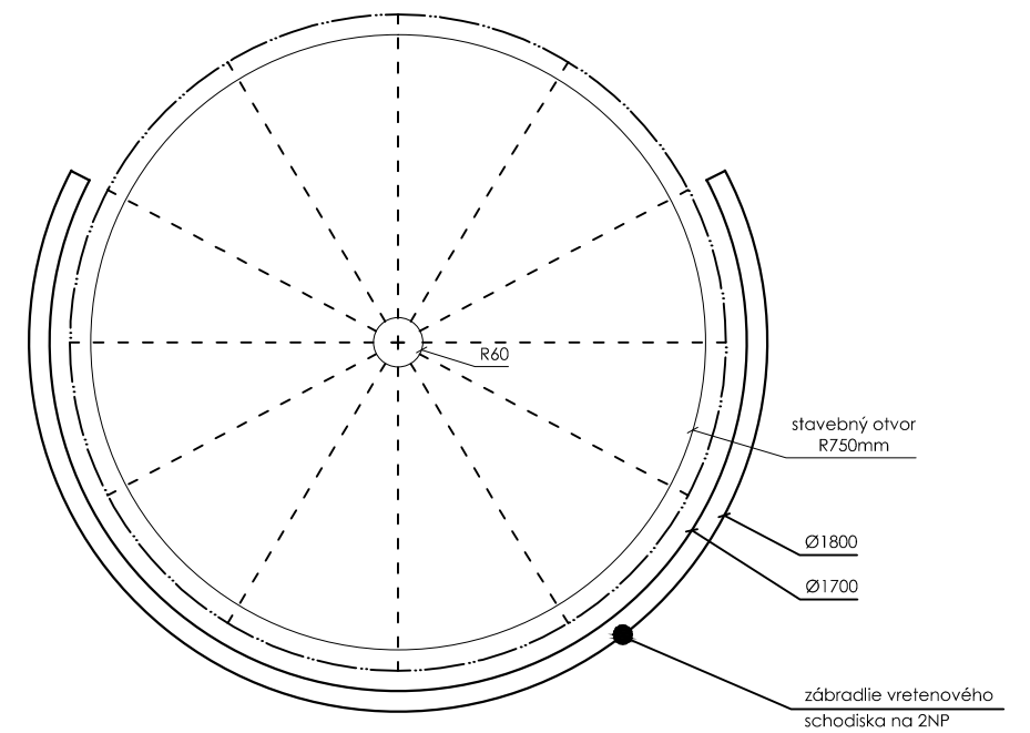
pôdorys - zábradlie vretenového schodiska 2NP
