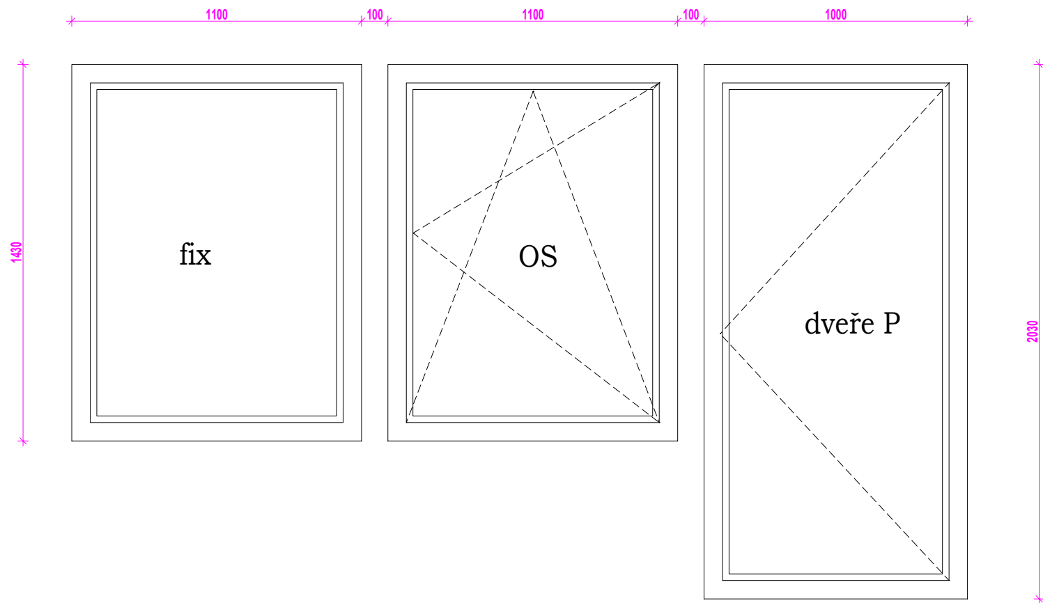
POHLED VNITŘNÍ
