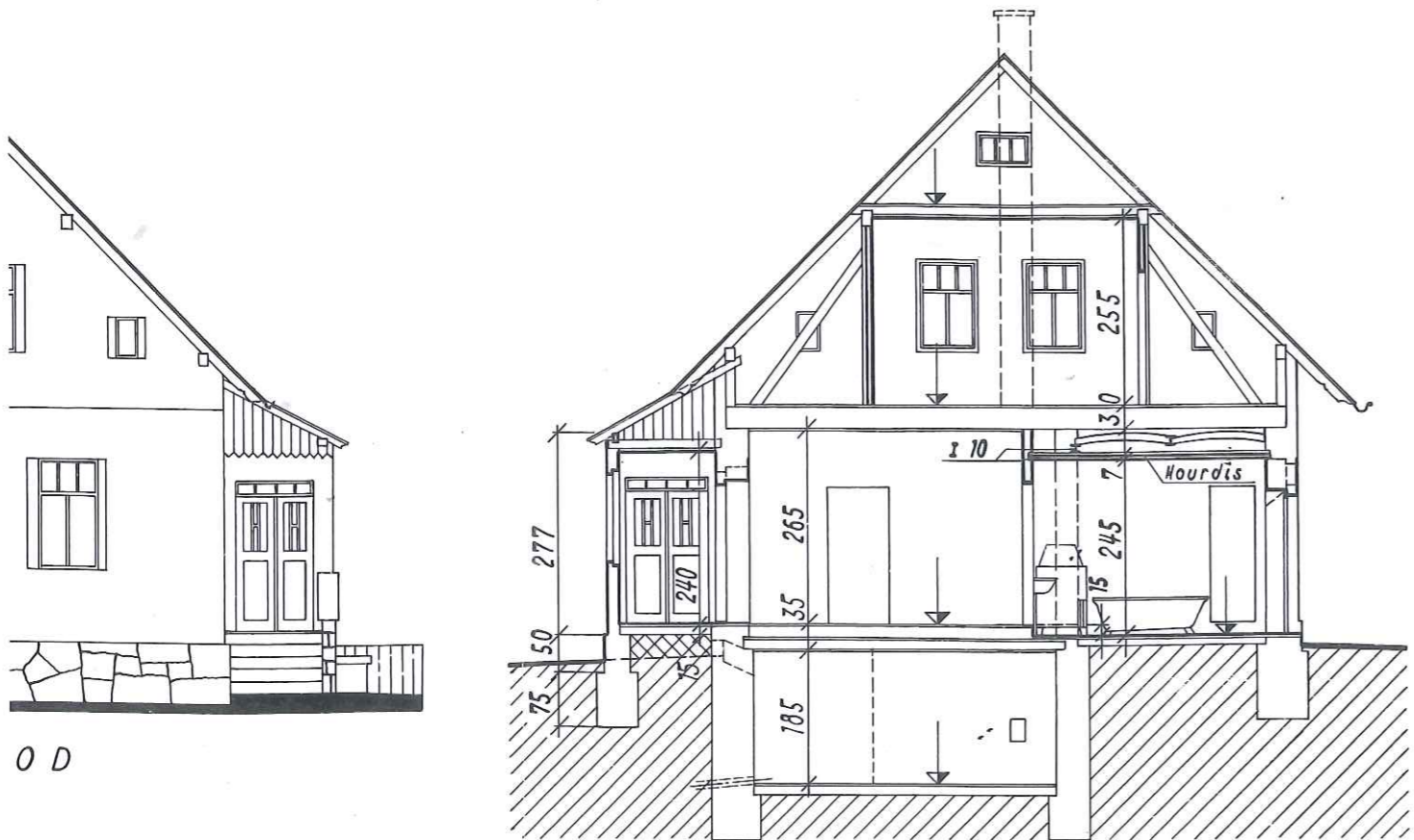
ŘEZ A-B
