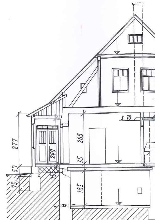
ŘEZ A-B
