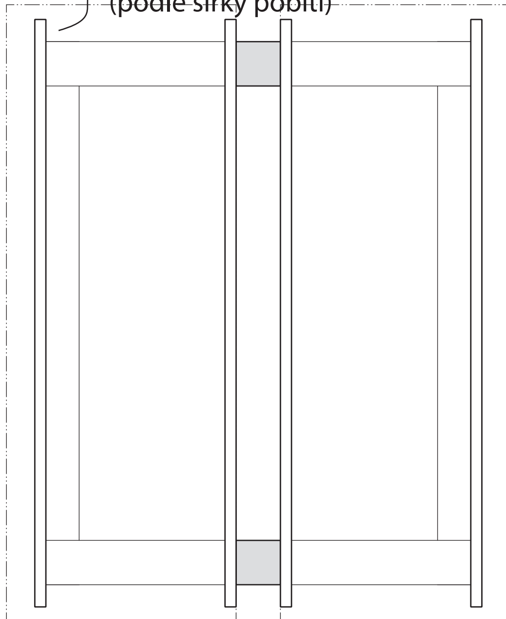
+ latě pro pobití „palubkama“
