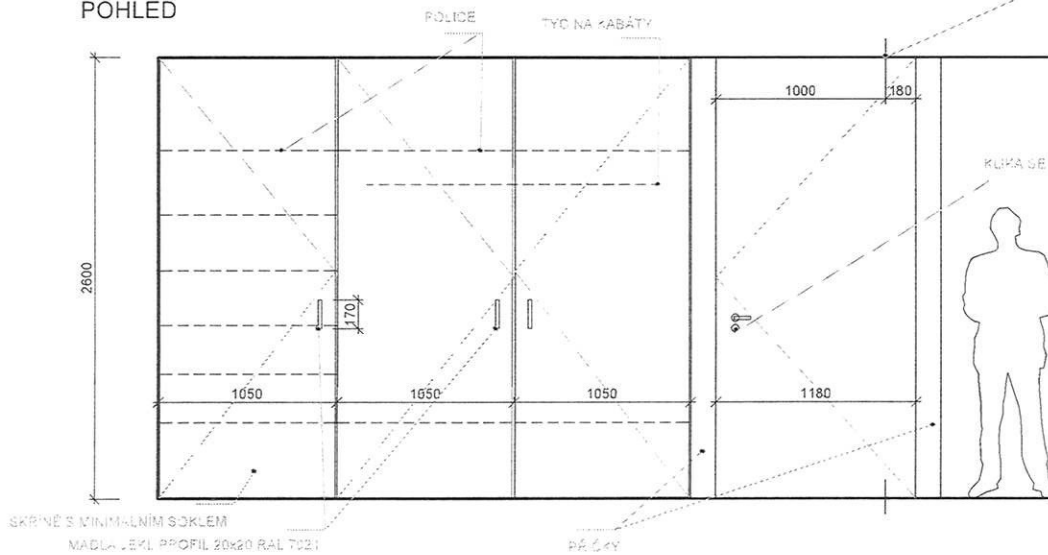
POHLED
