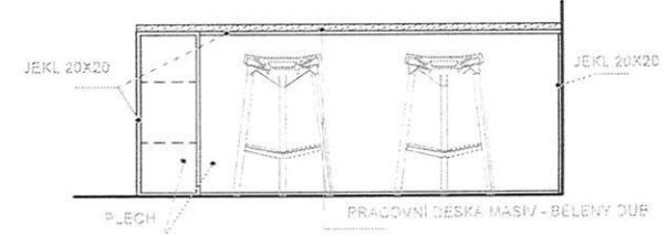
P4 - OSTRŮVEK
