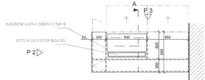
P2 - OSTRŮVEK
