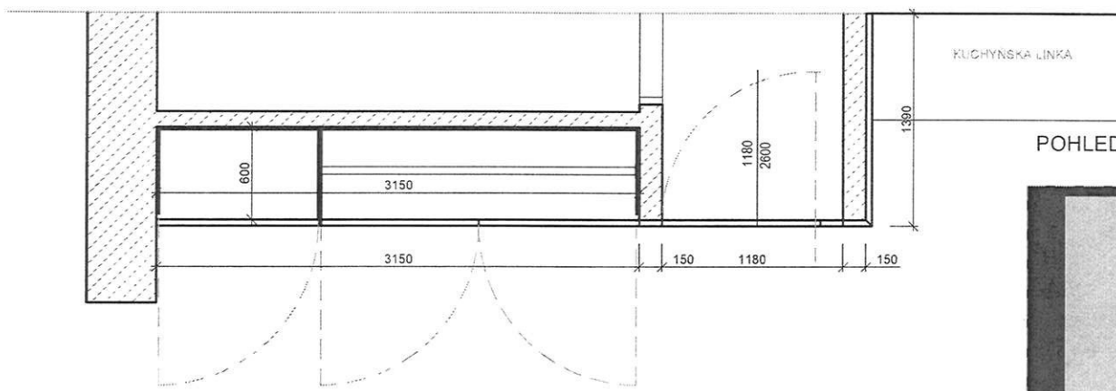
PŮDORYS
