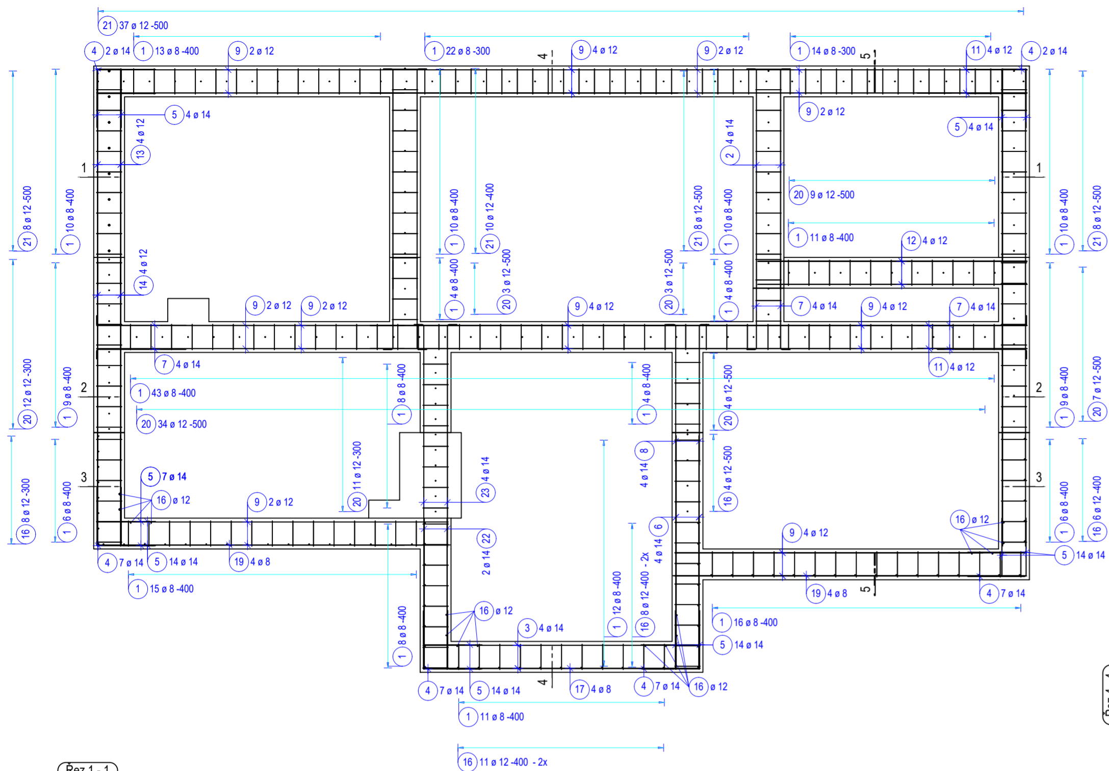
Řez 1-1
