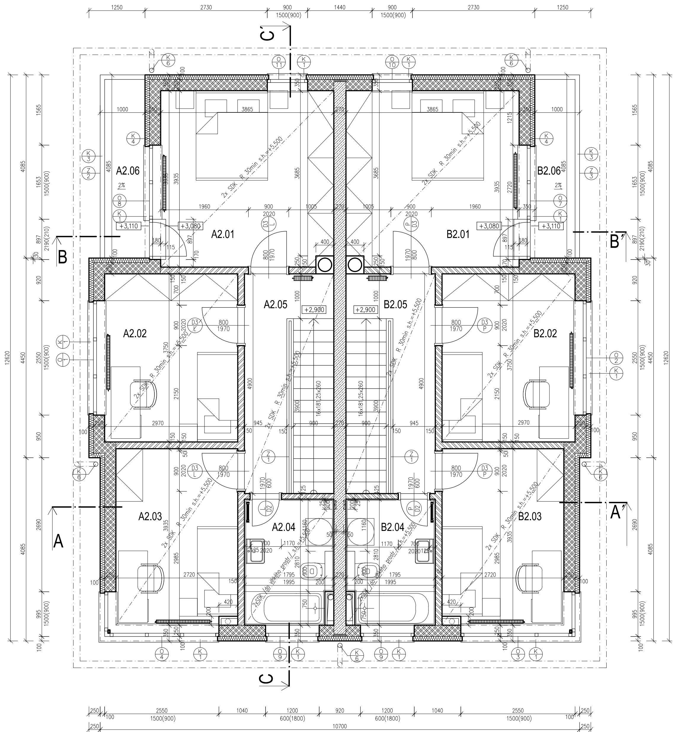
PÓDORYS 2.NP
