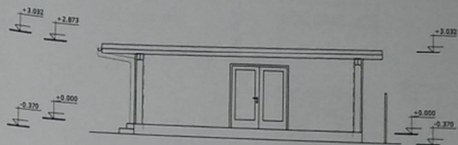
POHLED SEVEROVÝCHODNÝ
