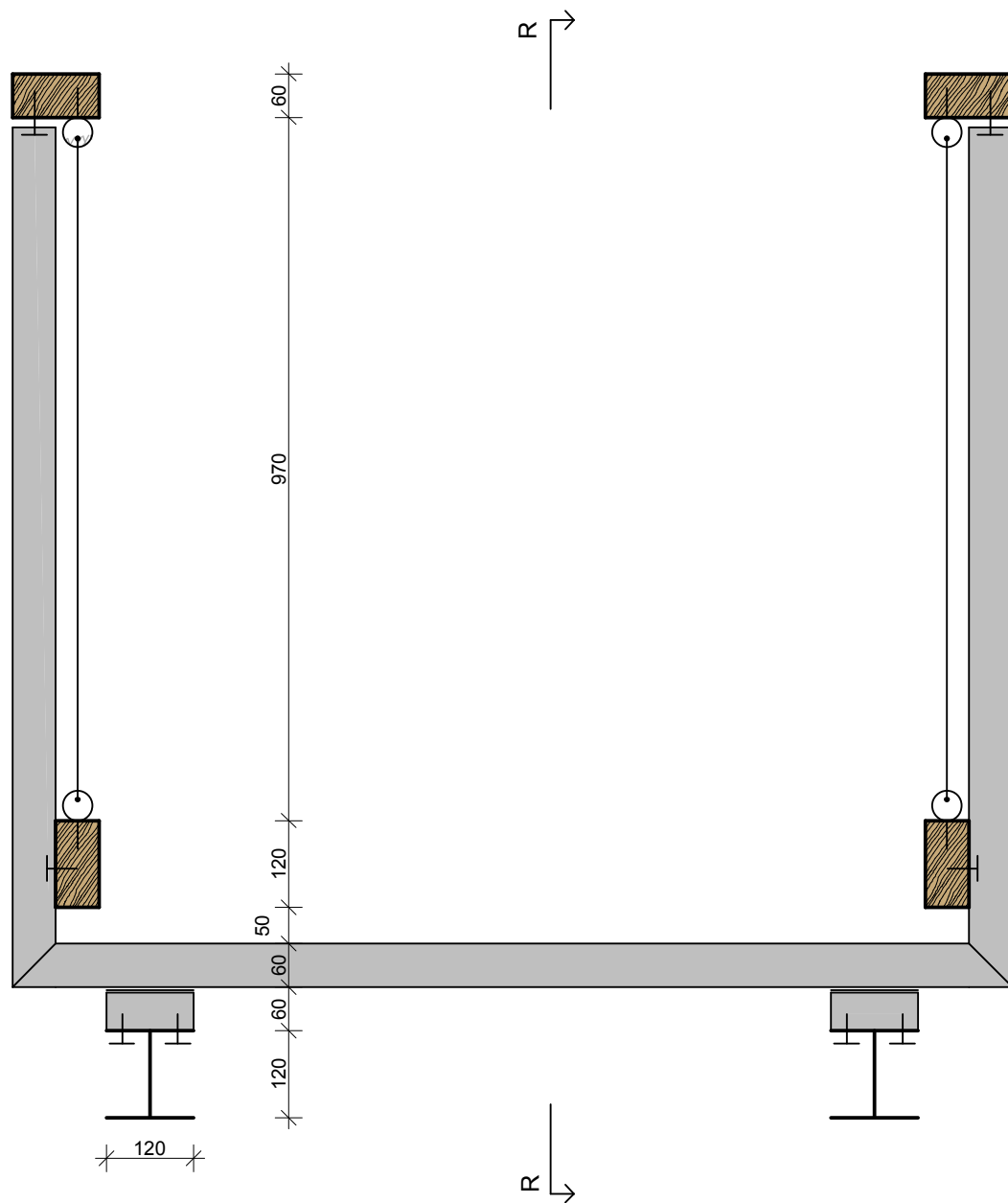
PRIEČNY REZ
