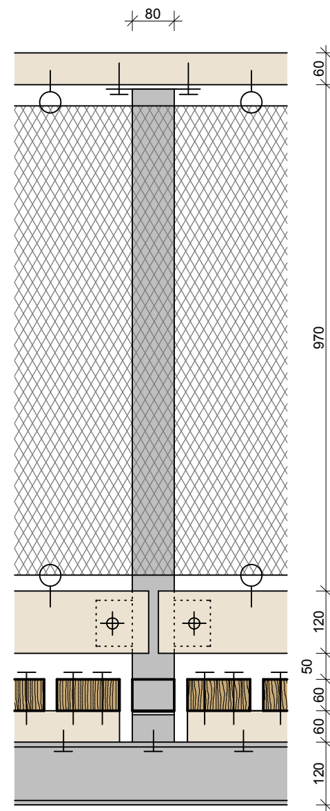
POZDĽŽNY REZ R-R
