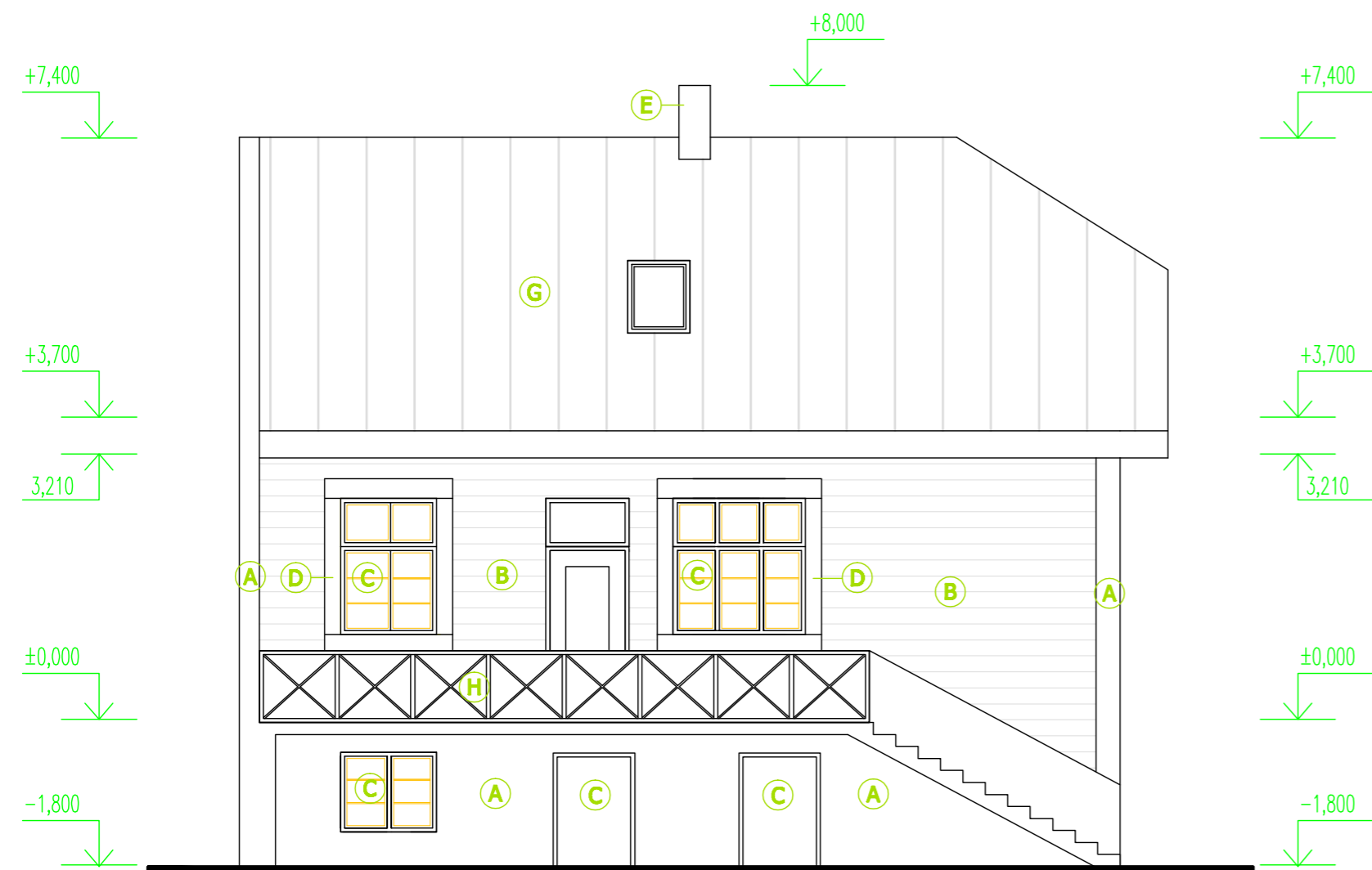
POHĽAD JUŽNÝ
