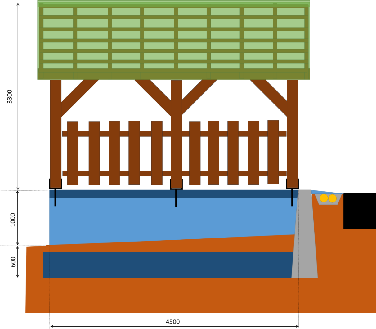
Bočný pohľad
