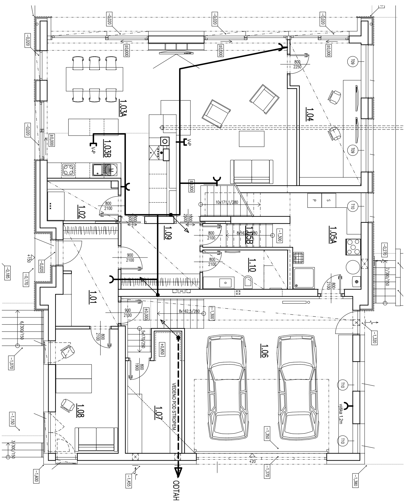
PŮDORYS 1.NP ÚROVEŇ ±0,000
