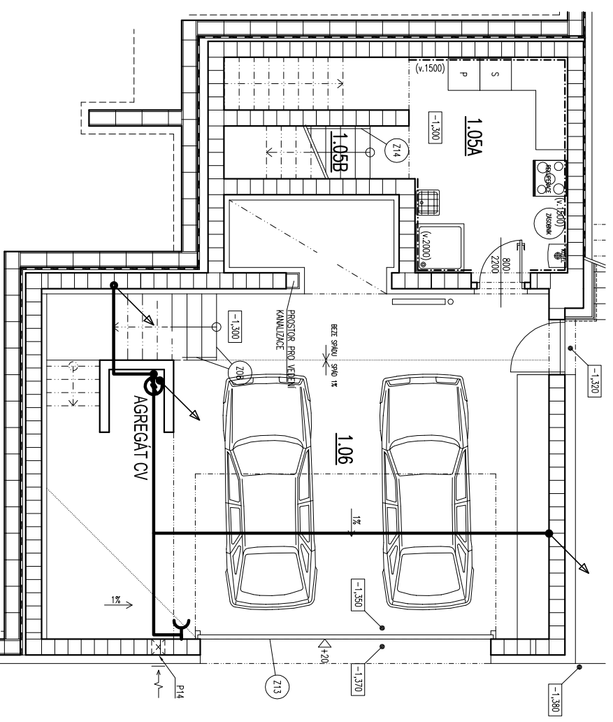
PŮDORYS 1.NP ÚROVEŇ -1,300
