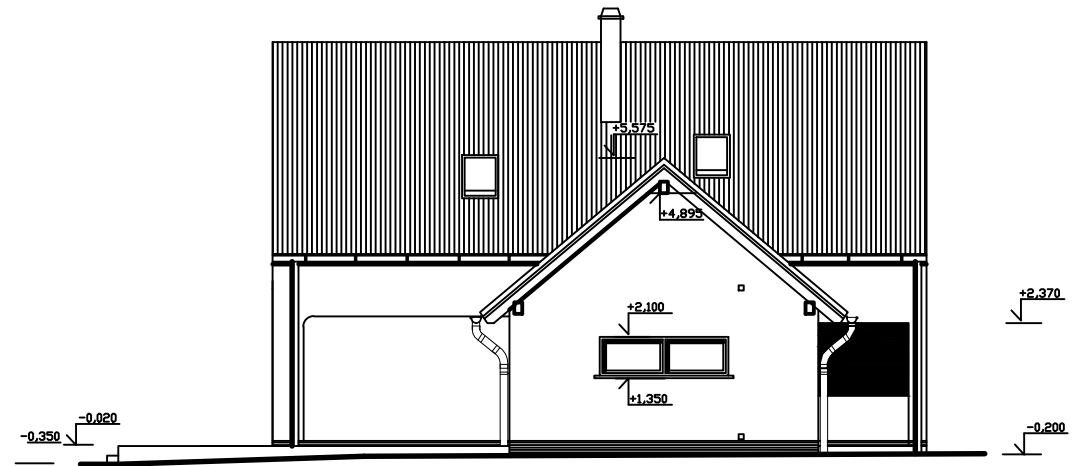
POHLED BOČNÍ
