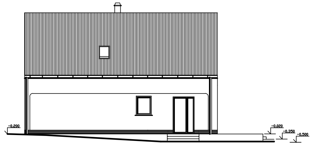
POHLED BOČNÍ
