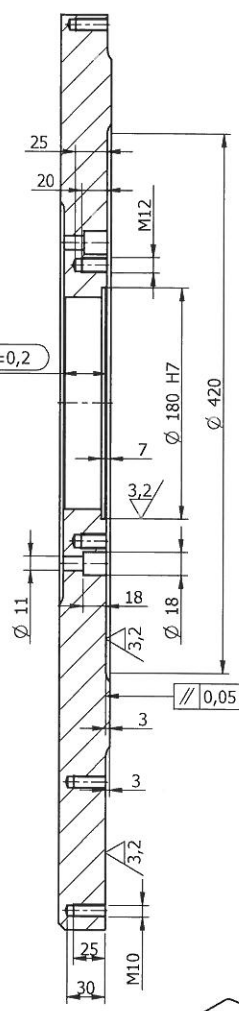
B-B 1:2
