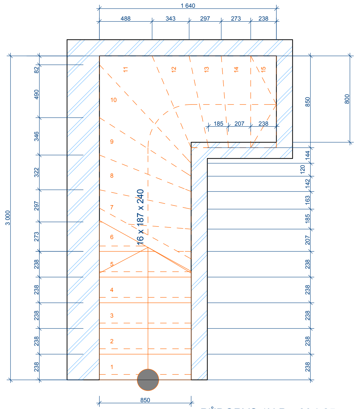
PŮDORYS 1N.P. - M 1:25
