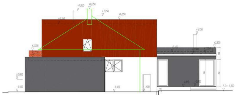
POHLED JUHOVÝCHODNÝ
