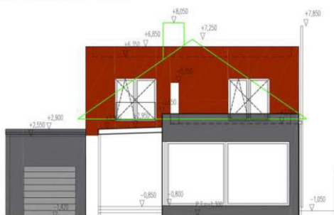
POHLED JUHOZÁPADNÝ - ULIČNÝ
