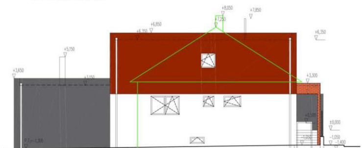
POHLED JUHOVÝCHODNÝ
