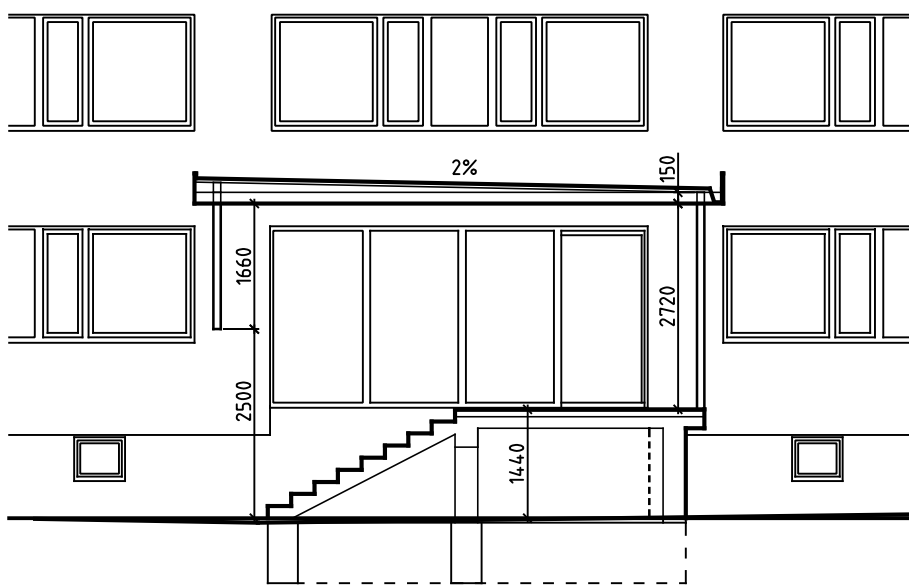
Podélný řez
