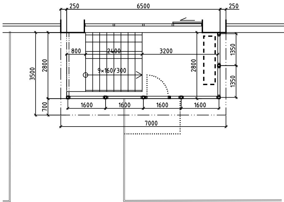
Půdorys
