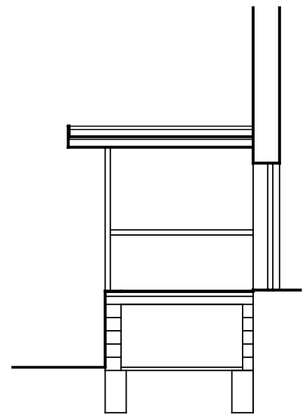
Příčný řez
