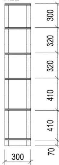
ŘEZ
