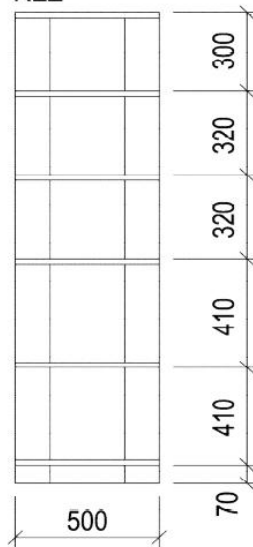
ŘEZ
