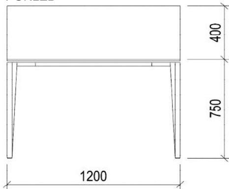
POHLED
