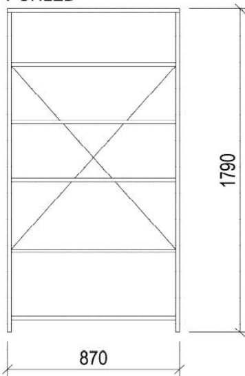
POHLED
