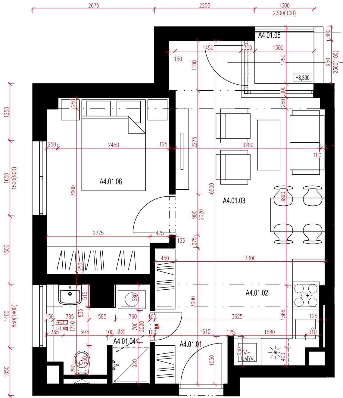
BYT A4.01
