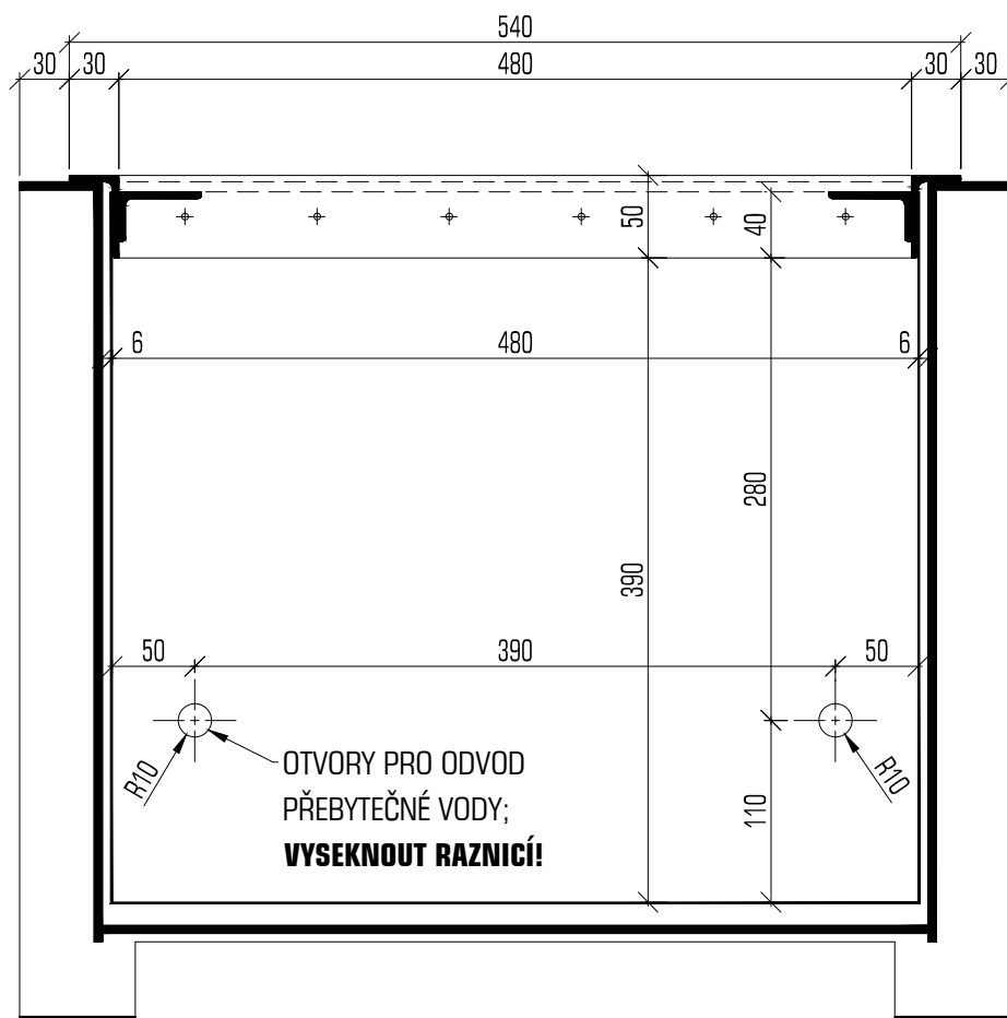
CELKOVÝ SVISLÝ ŘEZ A-A
