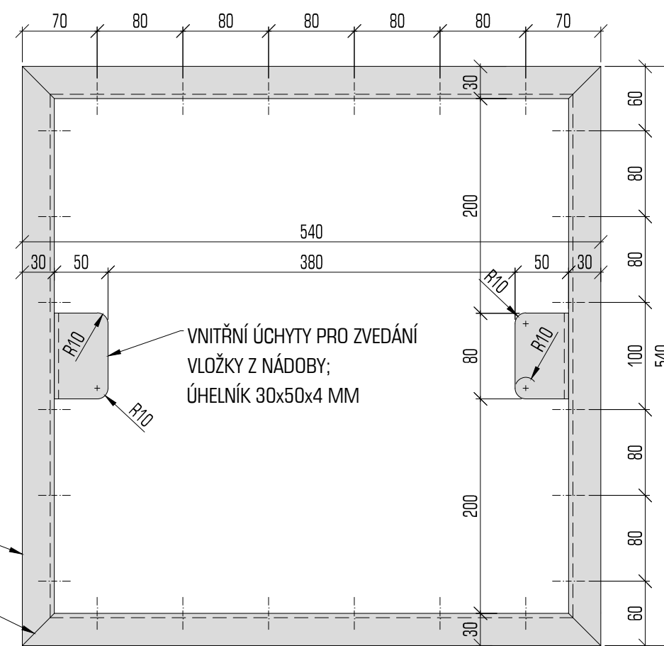
PŮDORYSNÝ POHLED NA VLOŽKU
