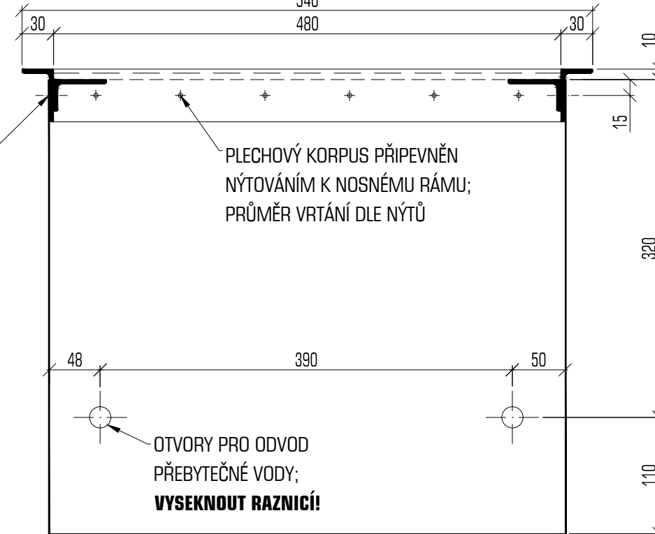
SVISLÝ ŘEZ VLOŽKOU A-A
