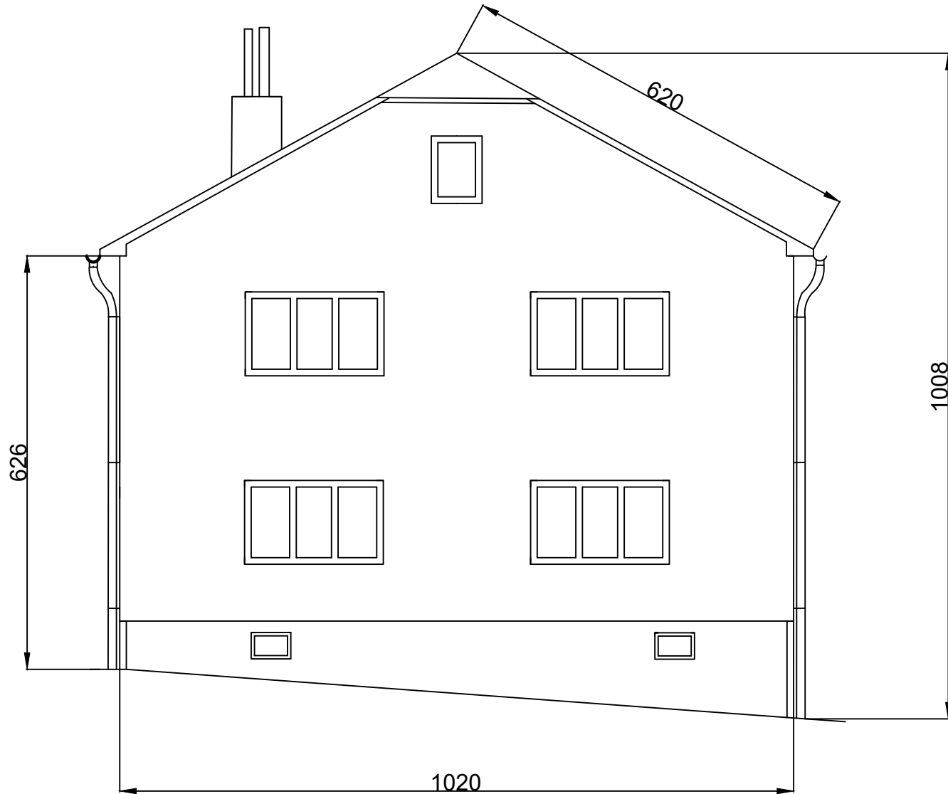
Pohled západní
