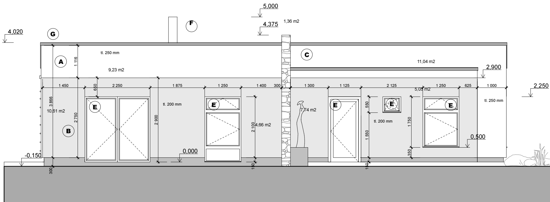
Pohled jižní
