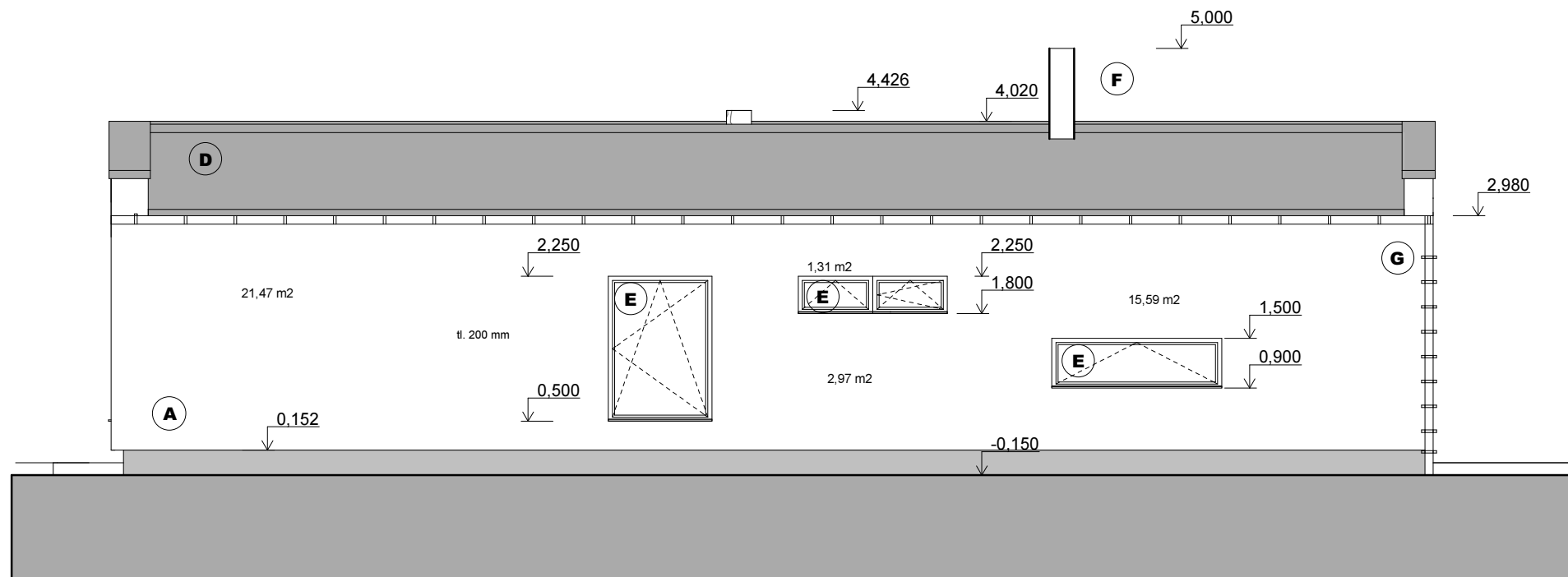
Pohled severní
