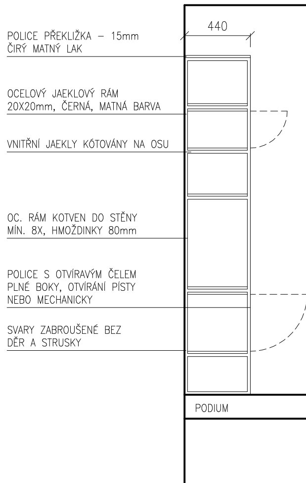
boční pohled
