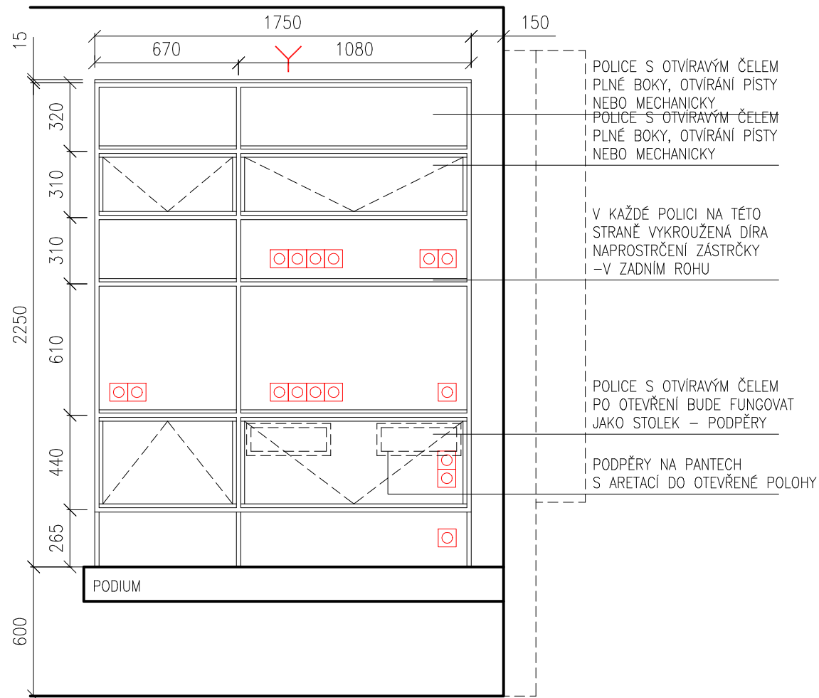
čelní pohled
