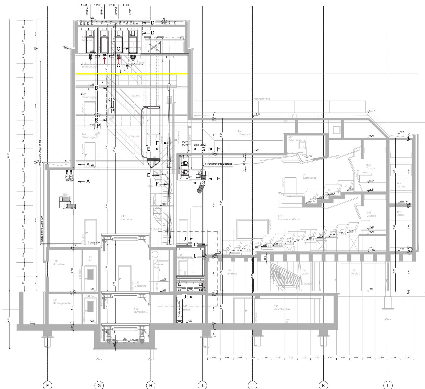
Längsschnitt F - F
