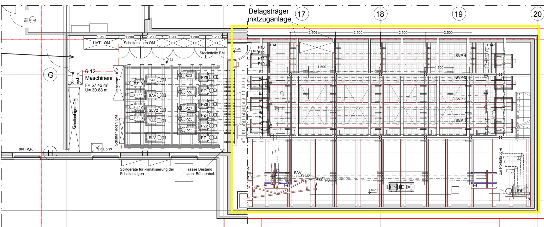
Grundriss Maschinenraum +13,35m / Grundriss Schnürboden +16,15m
