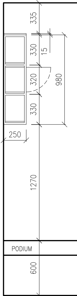
boční pohled
