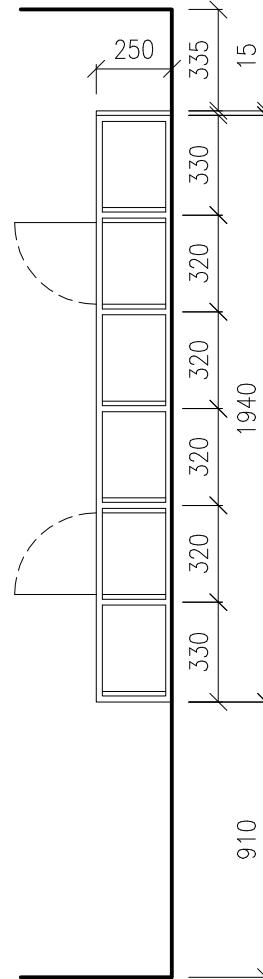
boční pohled
