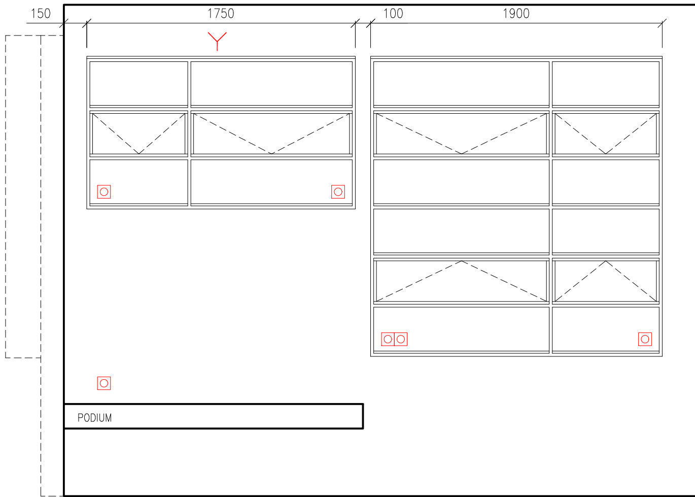
čelní pohled
