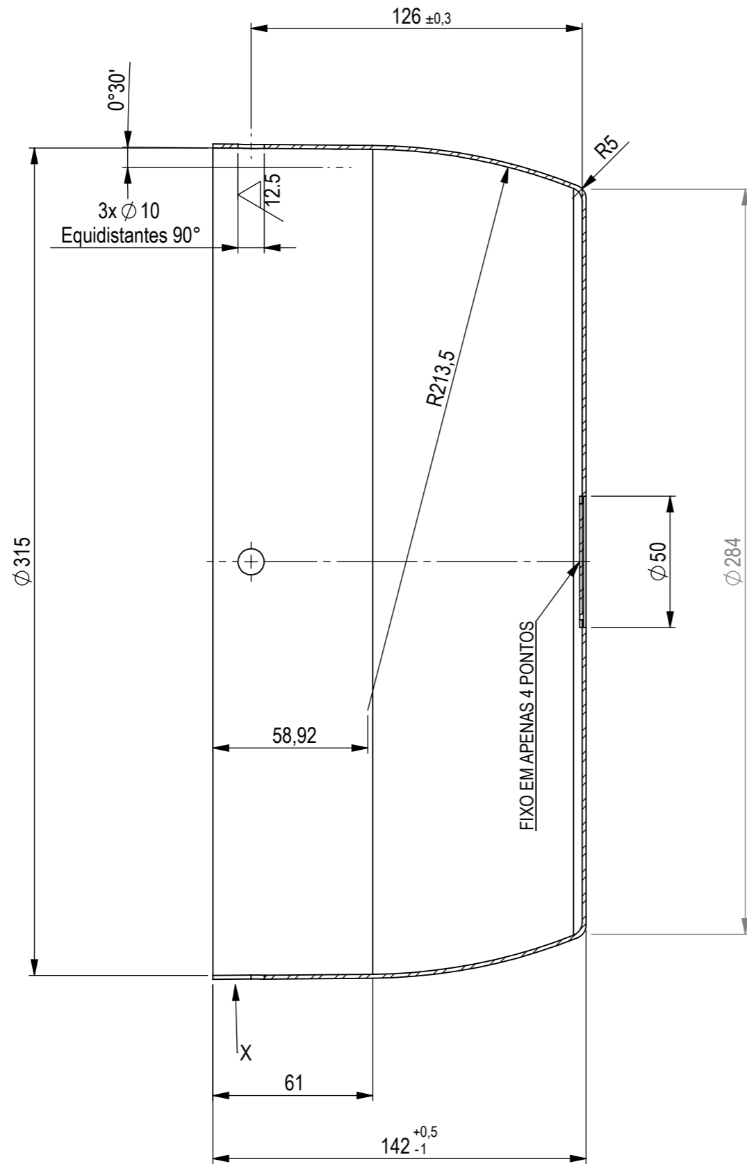
CORTE A-A ESCALA 1 : 2
