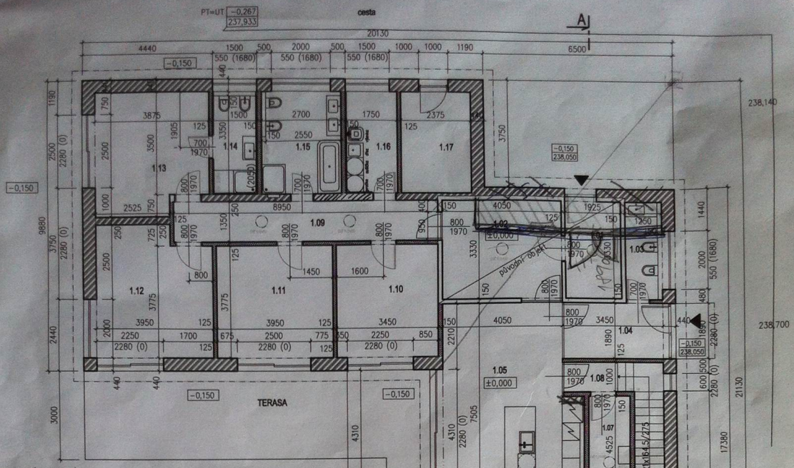
TABULKA MÍSTNOSTI
