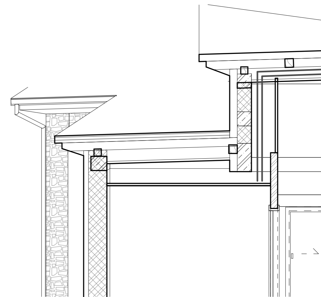
RIEŠENIE REKUPERAČIE - PRECHOD
