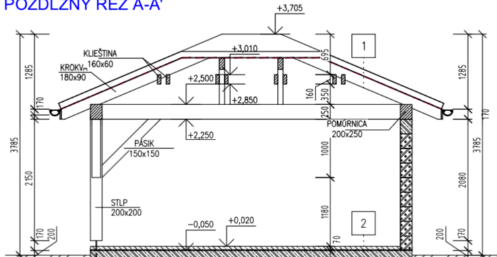
POZDĽŽNY REZ A-A'
