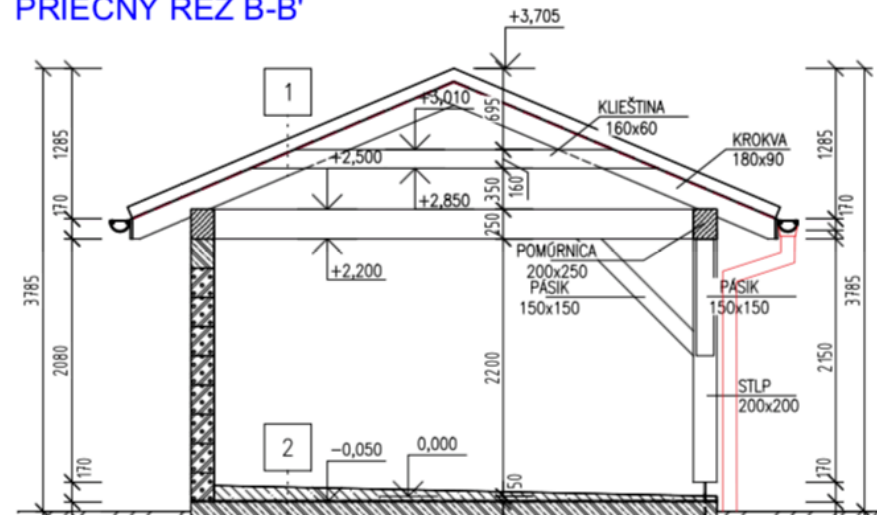
PRIEČNY REZ B-B'
