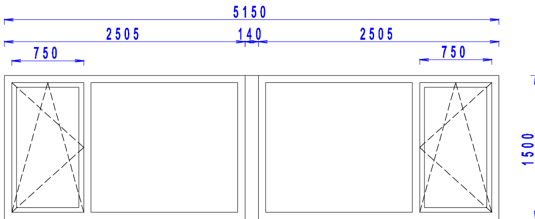
OKNO PLASTOVÉ ČÁSTEČNĚ OTVÍRAVÉ . . . . . 1ks
