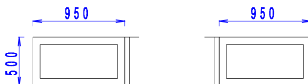
OKNO PLASTOVÉ NEOTVÍRAVÉ ROHOVÉ DVOUDÍLNÉ. . . 1ks
