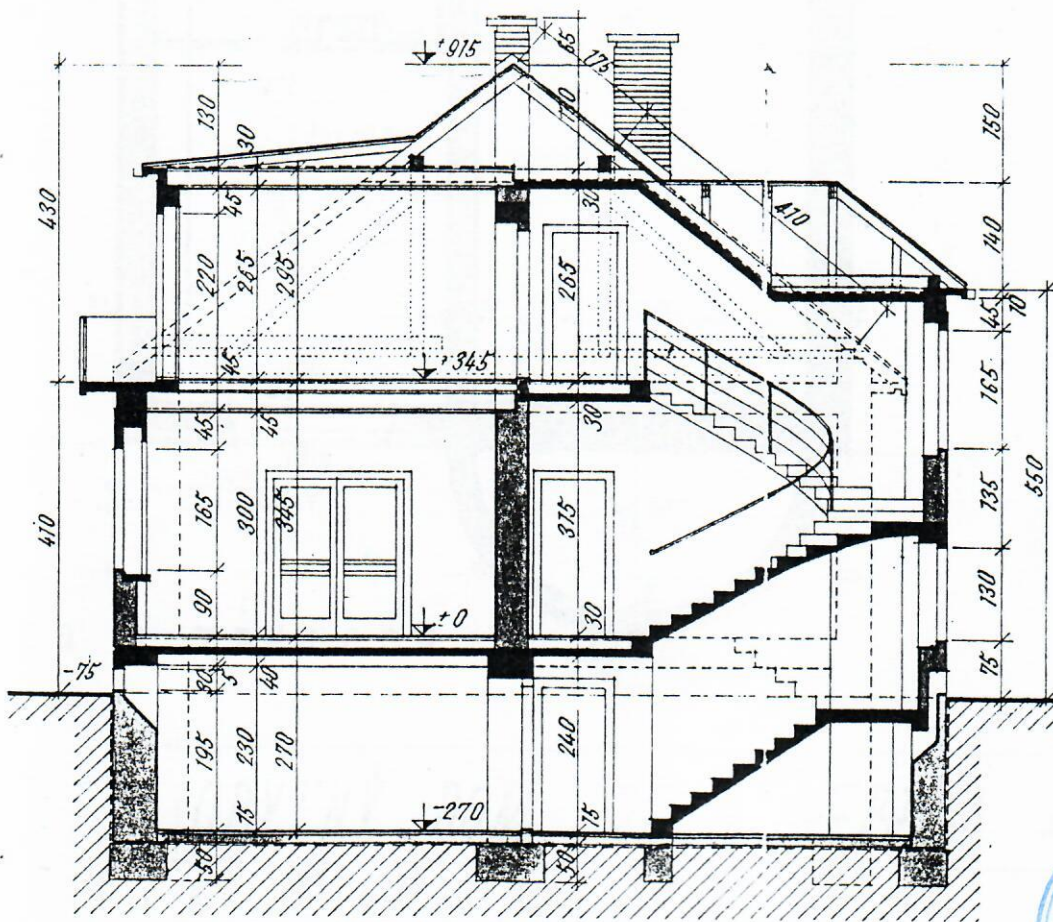
REZ PRIEČKY
