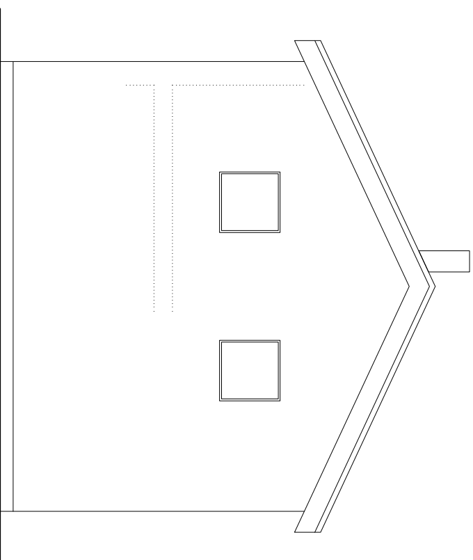
POHLED SEVERNÍ M 1 : 100
