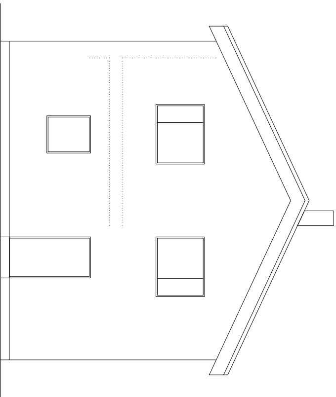
POHLED JIŽNÍ M 1 : 100
