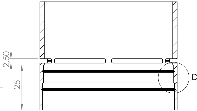
ŘEZ A-A
