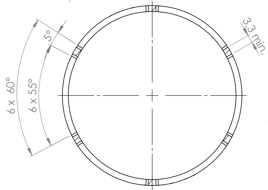
ŘEZ B-B
