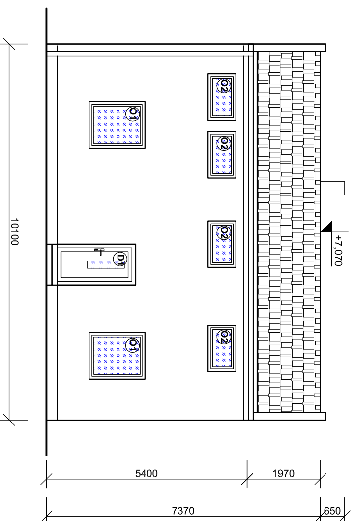
Pohled zahradní
