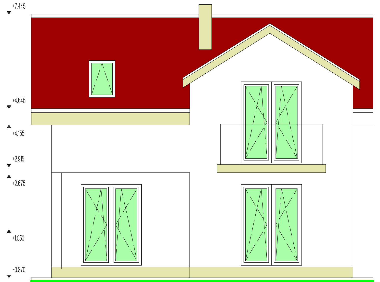
pohľad zadný
