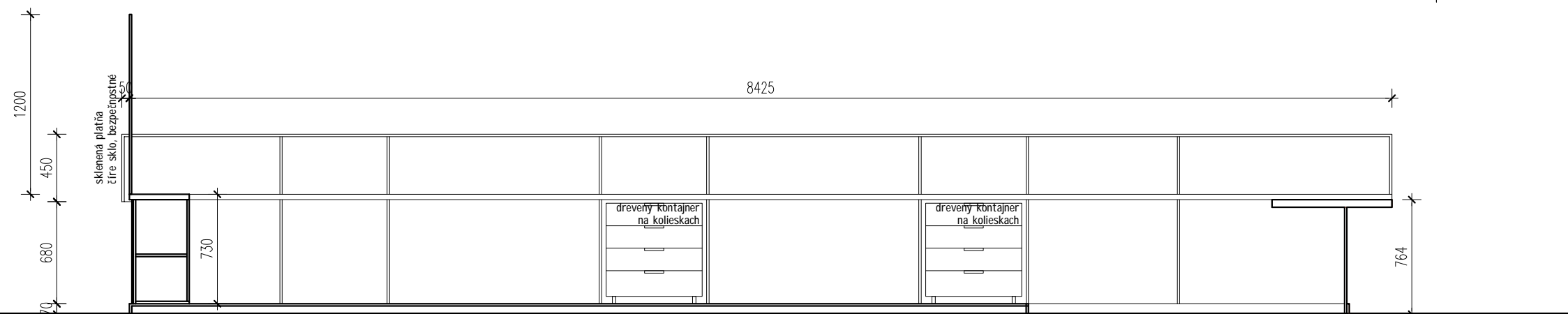
POHĽAD NA PULT Z VNÚTRA m=1:35
