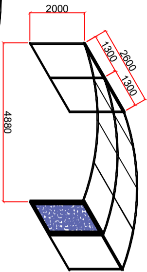
Zastřešení díl B I. jednostranně posuvný
