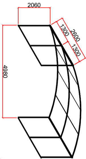
Zastřešení díl A III. jednostranně posuvný
