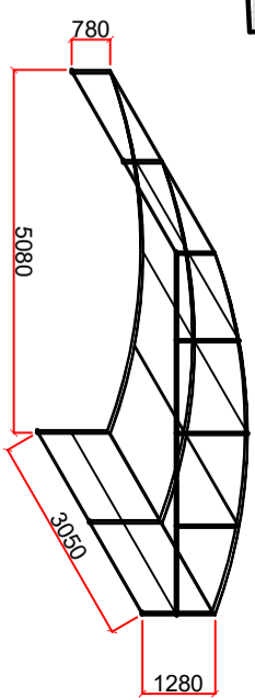
Zastřešení díl A II. pevný
