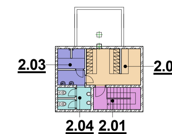
PŮDORYS 2NP - VSTAVBA
