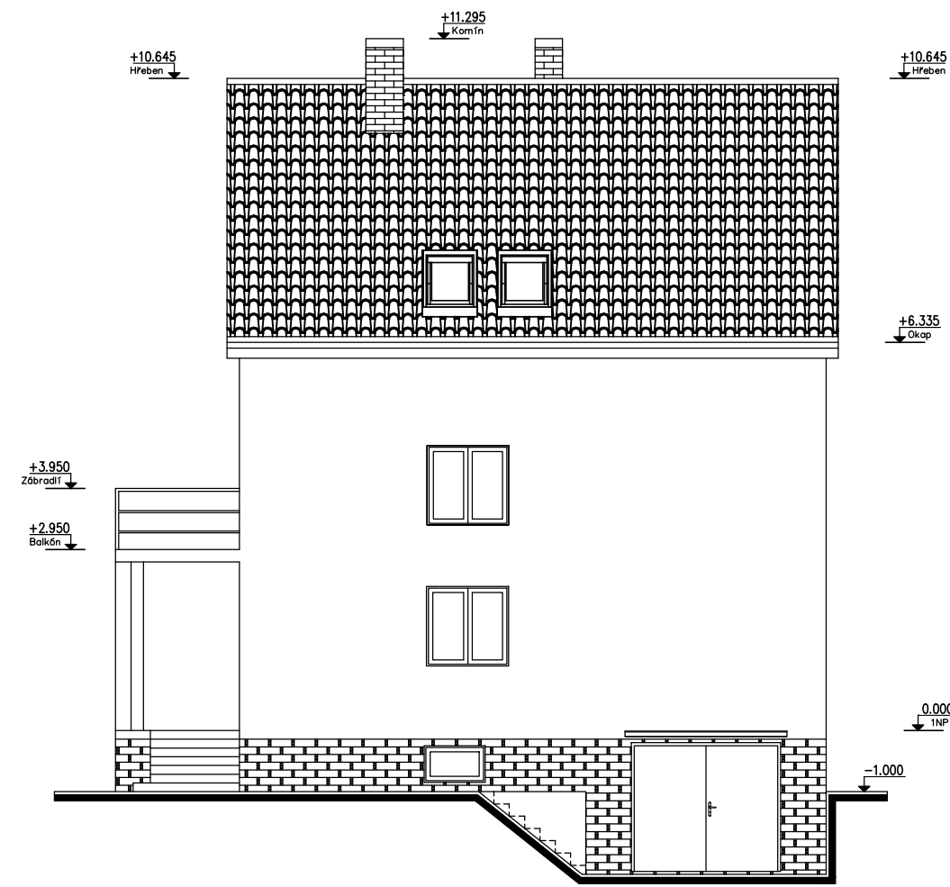
Pohled západní
