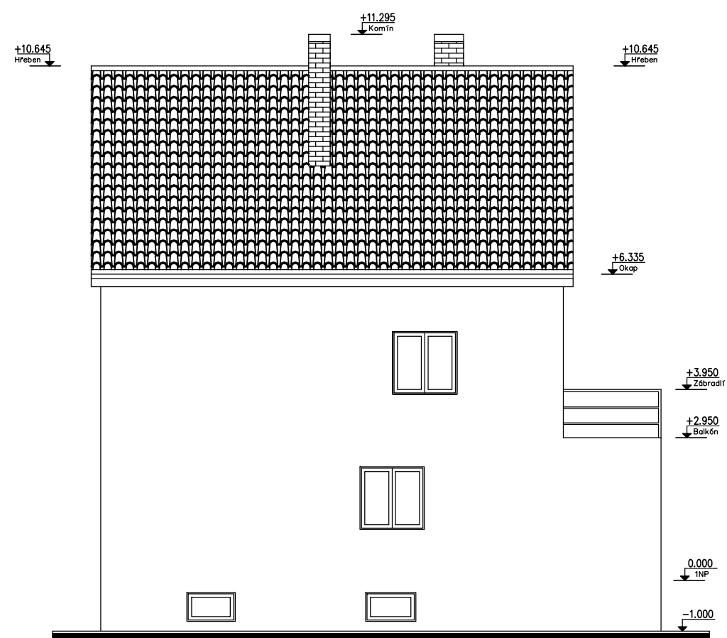
Pohled východní
