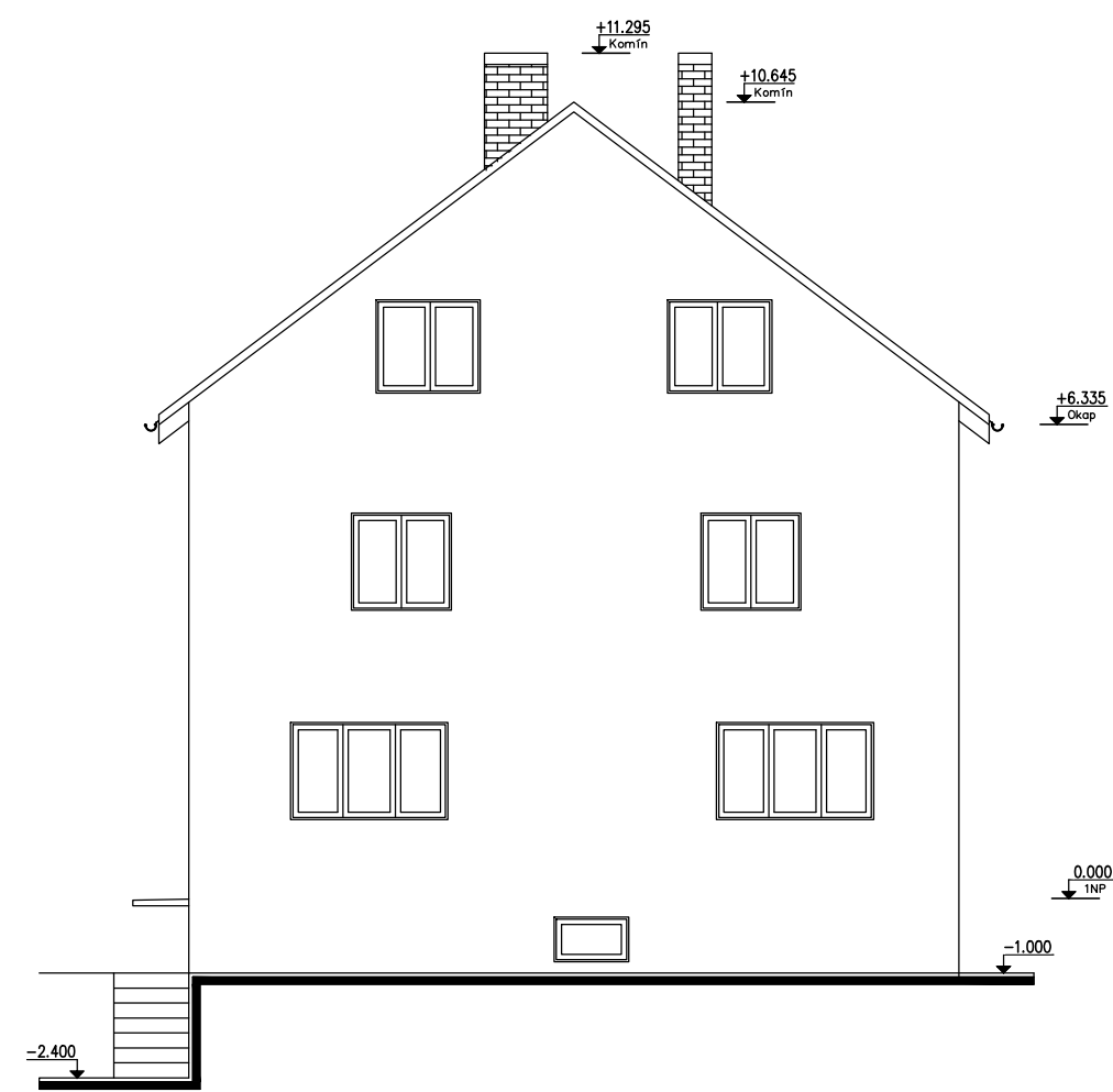
Pohled jižní
