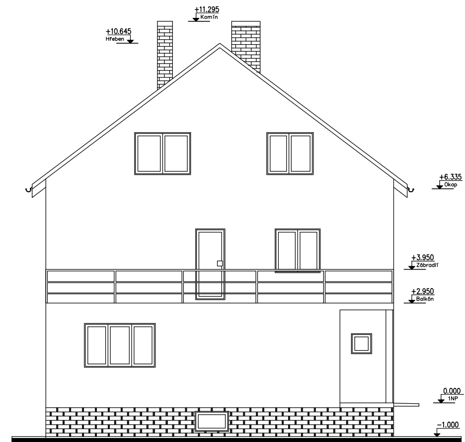
Pohled severní
