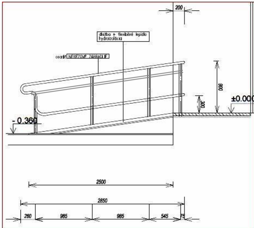
Tvar a rozmery zábradlia
