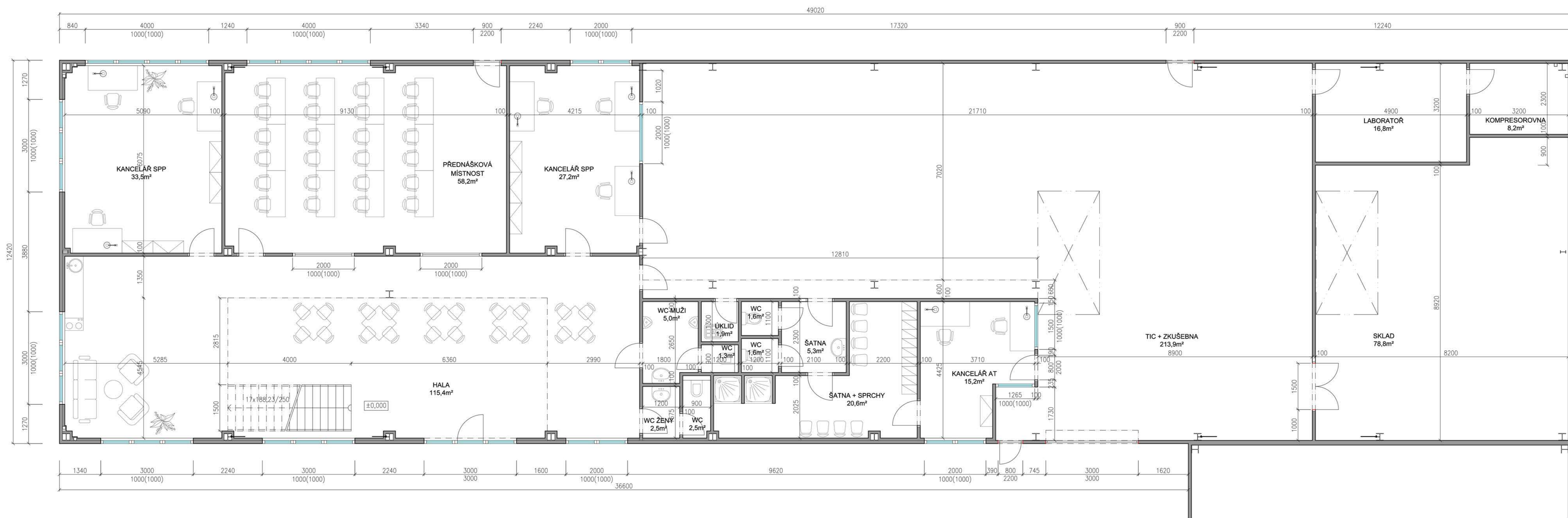
HALA RUDNÁ - VESTAVBA KANCELÁŘÍ PŮDORYS 1NP M - 1:50
