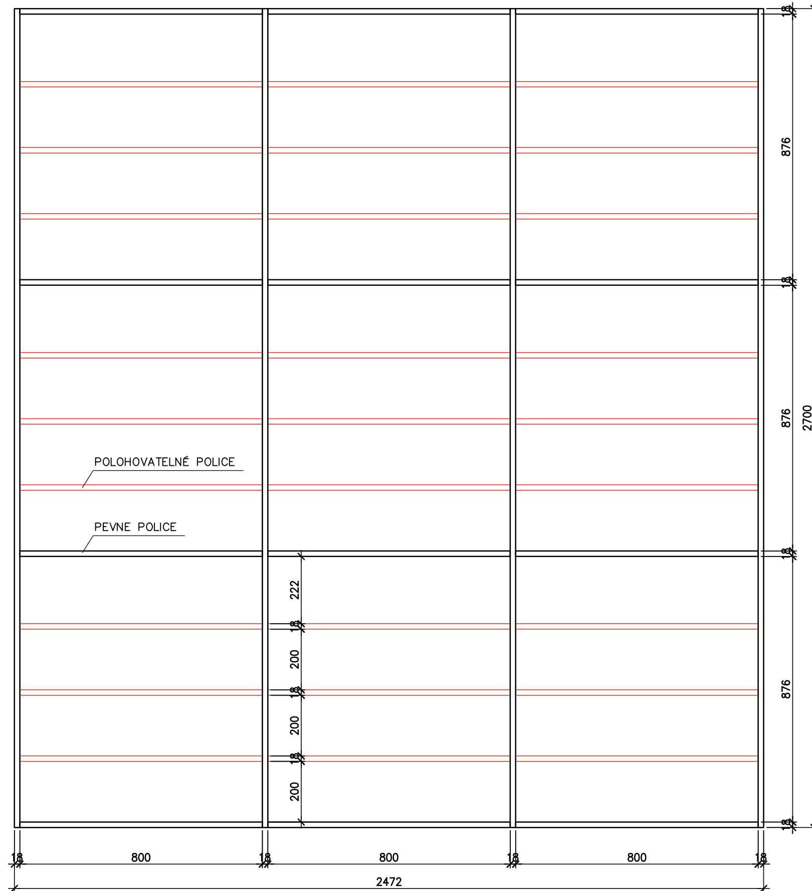
POHĽAD ČELNÝ
