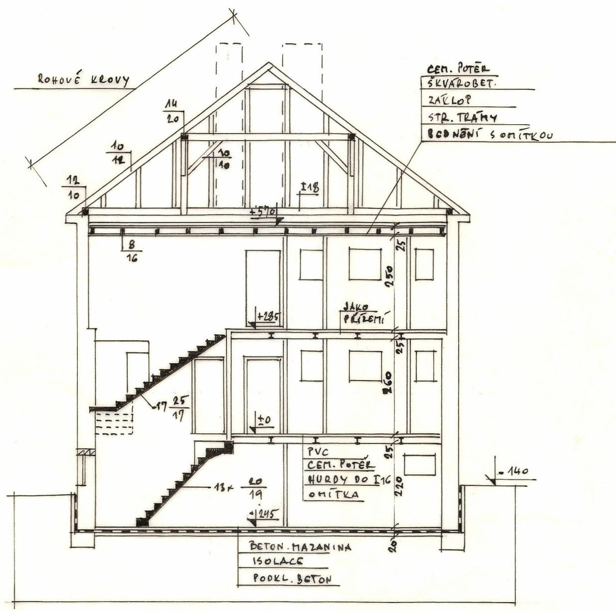
ŘEZ A-A'
