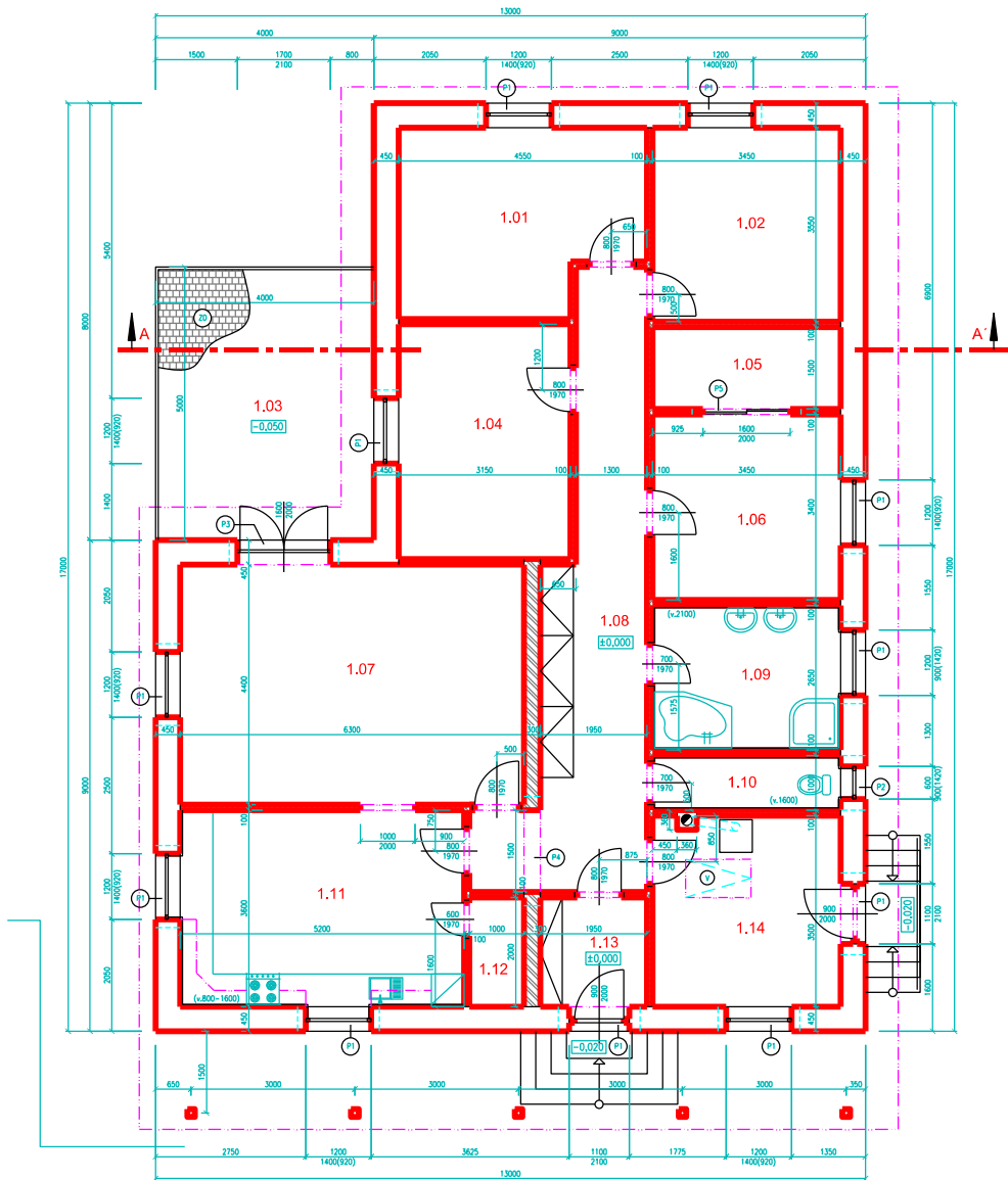
PŮDORYS 1.NP
